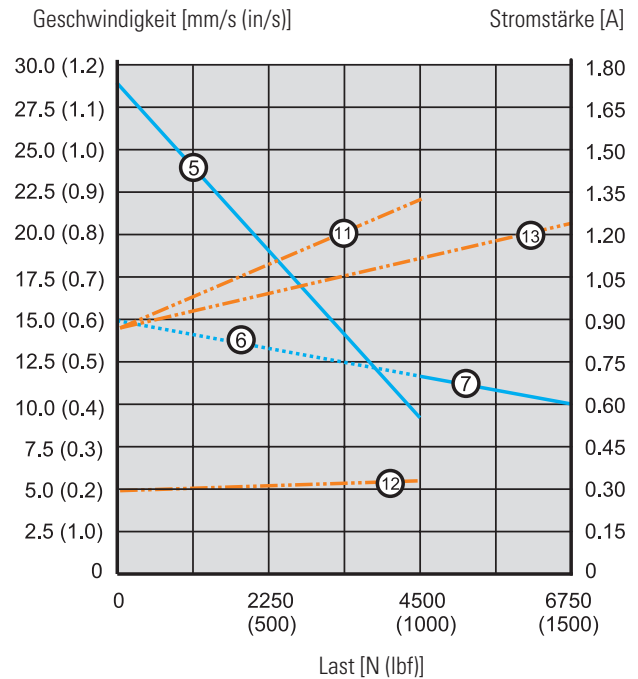
Geschwindigkeitskurven-Diagramm 2
